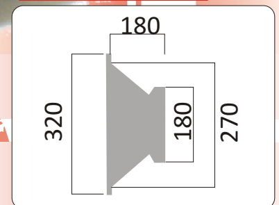
Dimensiones (mm)
